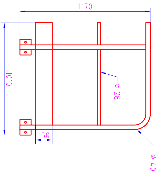
VOORRAANZICHT
